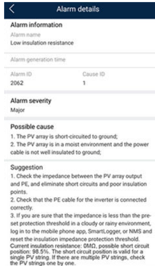
Figura E-1 Detalii despre alarmă
