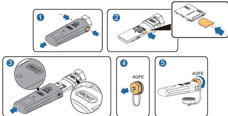
Figura 5-4 Instalarea unui 4G Smart Dongle
