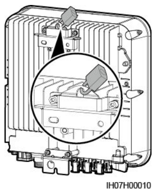
Figura 4-12 Instalarea unui sistem de blocare antifurt
